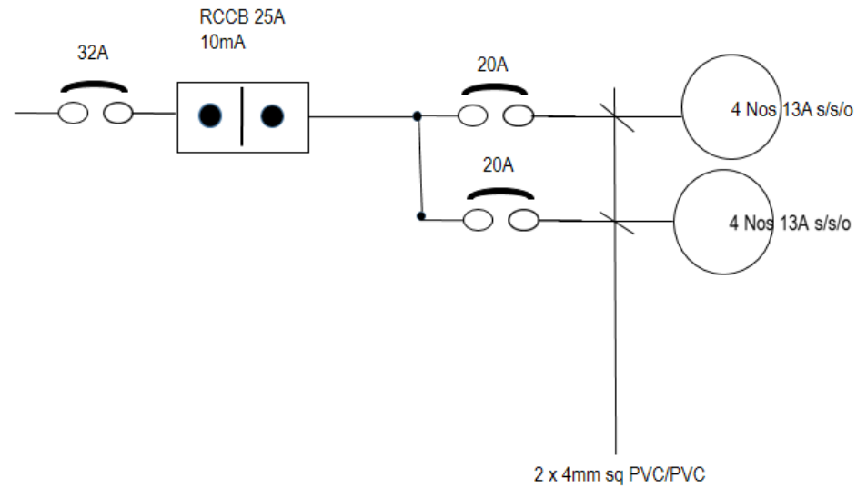
Lukisan Litar Extension dgn 8 keluaran mata kuasa
